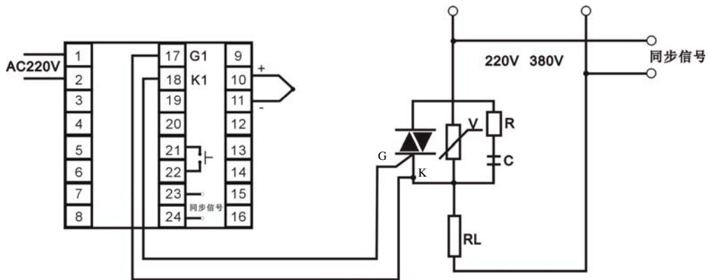
图 6.7 接双向可控硅（采用负脉冲触发）
