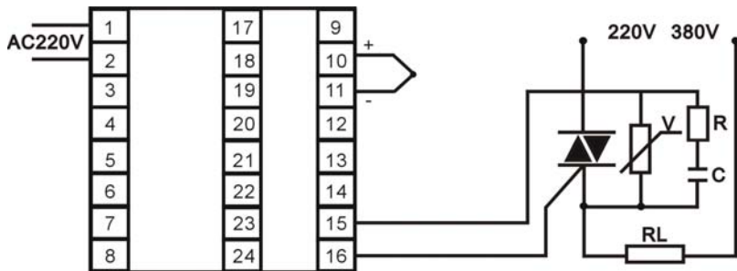
图 6.1 接双向可控硅
