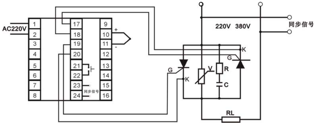
图 6.8 接单向可控硅反并联
