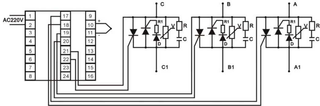
图 6.12 单向可控硅反并联
