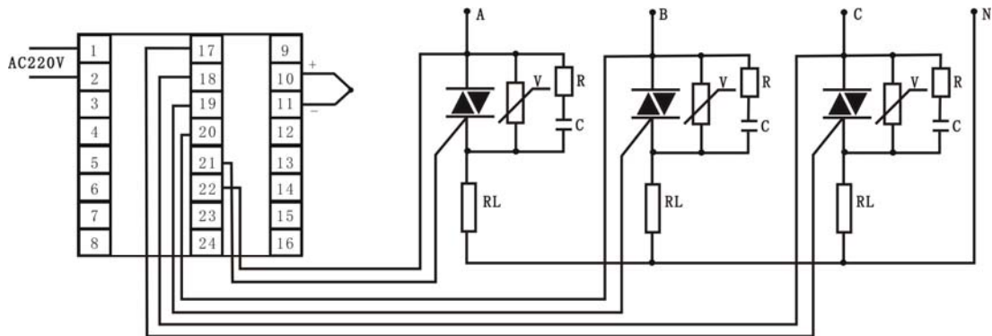
图 6.9 接双向可控硅
