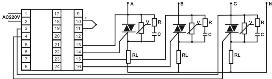
图 6.3 接双向可控硅
