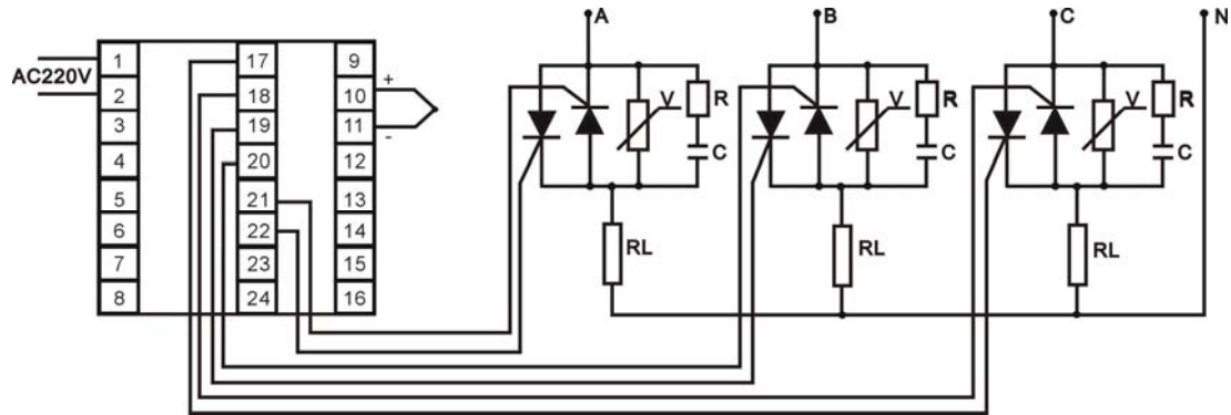
图 6.10 接单向可控硅反并联
