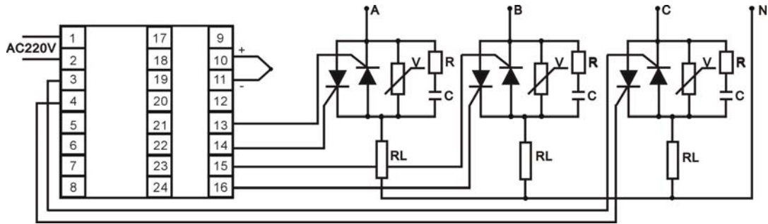
图 6.4 接单向反并联可控硅
