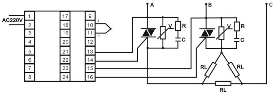
图 6.6 接双向可控硅、负载为 \Delta 型不接零线
