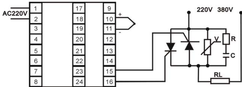
图 6.2 接两个单向可控硅
